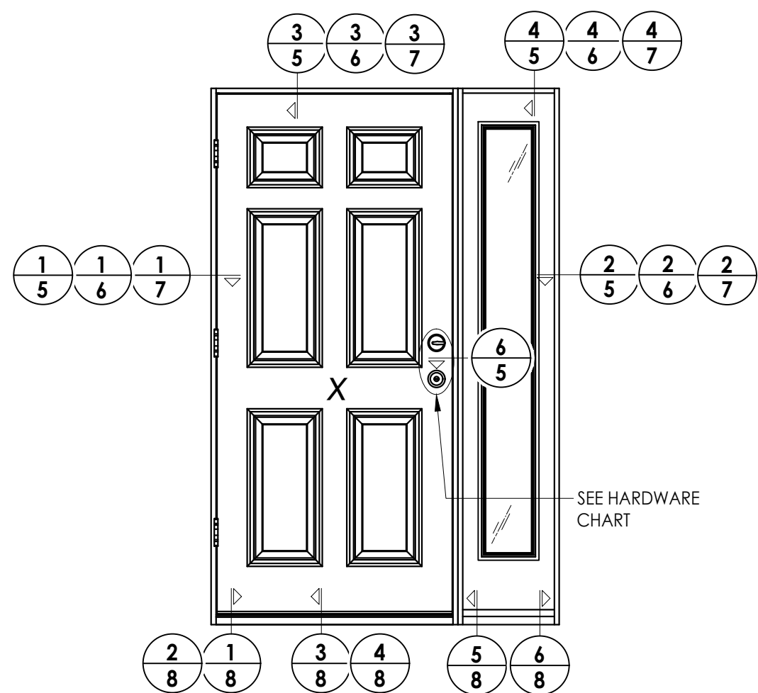
ELEVATION XO
