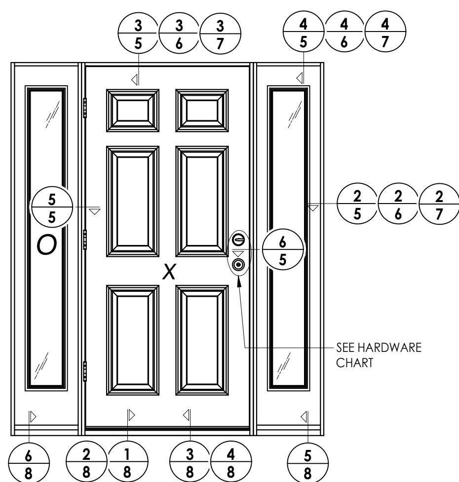
ELEVATION OXO
